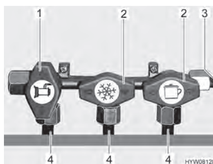
Bilde 95 Posisjon gassavstengingsventiler (eksempel)
