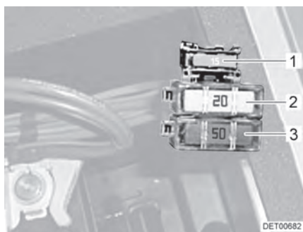
Bilde 101 Sikringer ved startbatteriet
