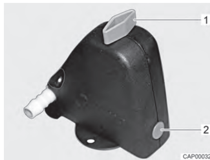
Bilde 131 Sikkerhets-/avtappingsventil lukket
