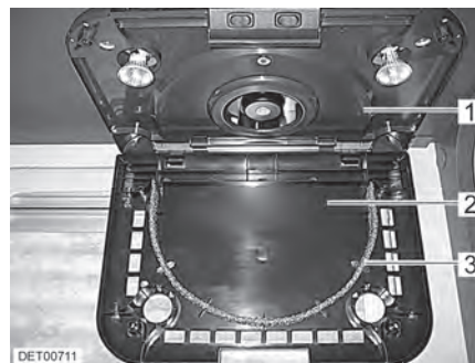
Bilde 147 Ta ut fettfilteret
