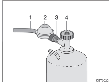
Bilde 93 Tilkobling gassflaske
