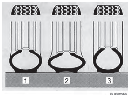
Bilde 160 Dekkets anleggsflate
