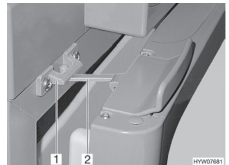
Bilde 125 Kjøleskapsdør i luftestilling (Thetford)
