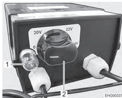
Bilde 114 Bryter for elektrisk gulvvarme
