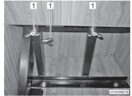
Bilde 18 Setesokkelen sikres med vingemuttre
