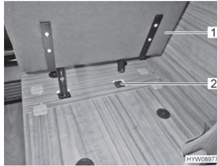
Bilde 17 Setesokkelen plasseres i holderen
