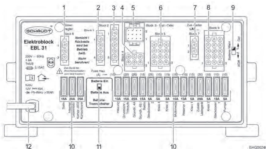
Bilde 96 Strømsentral (EBL 31)
