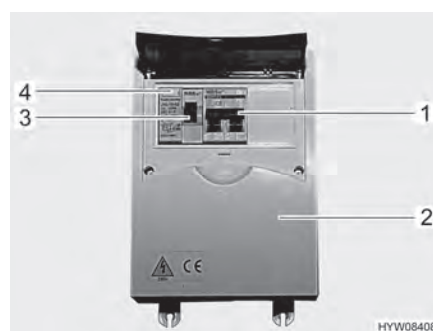
Bilde 98 230 V-sikringsboks med ledningsbeskyttelsesbryter og FI-bryter
