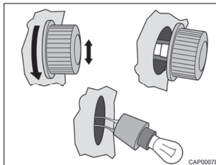
Bilde 151 Retningsviser på siden (12 V/5 W)
