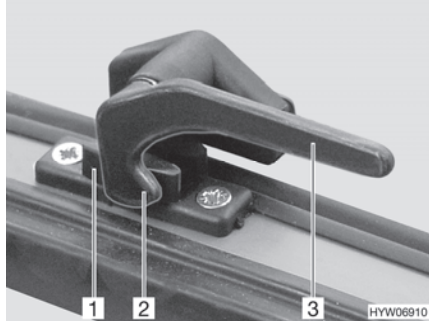
Fig. 43 Palanca de bloqueo en la posición "cerrada"
