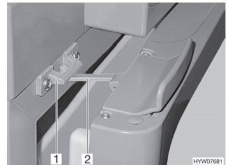
Fig. 130 Puerta del frigorífico en posición de ventilación (Thetford)
