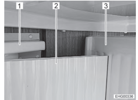
Fig. 146 Posición correcta de la pared giratoria pequeña
