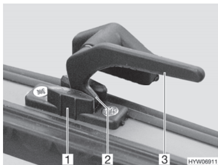
Fig. 45 Palanca de bloqueo en la posición de "ventilación continua"
