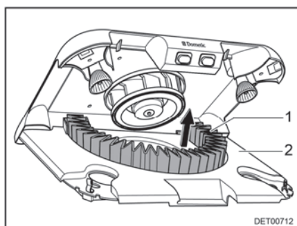
Fig. 153 Cambio del filtro de carbón activado
