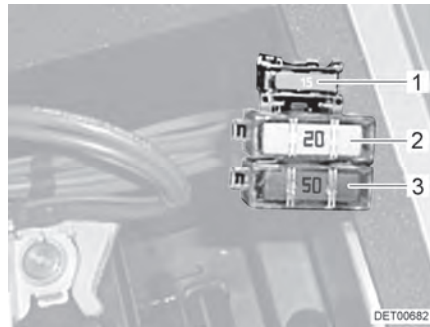
Fig. 100 Fusibles en la batería del motor de arranque sin amplificador de carga
