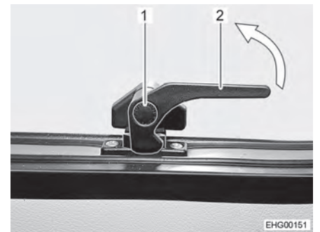
Fig. 37 Palanca de bloqueo inferior (posición "cerrada")
