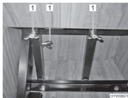
Fig. 17 Retener el asiento de enchufe con tuercas de mariposa
