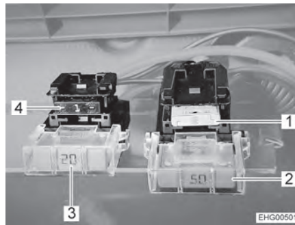
Fig. 103 Fusibles en la batería del habitáculo con amplificador de carga
