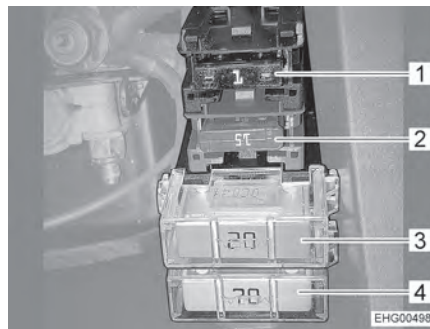
Fig. 101 Fusibles en la batería del motor de arranque con amplificador carga
