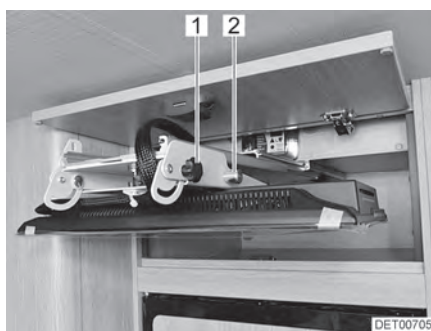
Fig. 63 Pantalla plana en el compartimento de televisor
