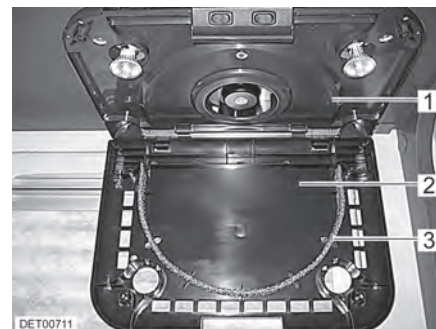
Fig. 152 Sacar el filtro de grasa
