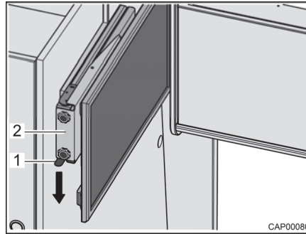
Fig. 67 Dispositivo de extracción con pantalla plana
