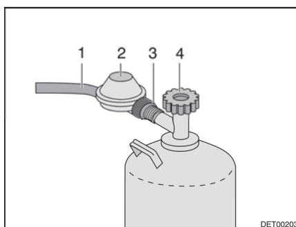
Fig. 91 Conexión de la bombona de gas
