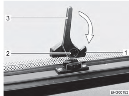
Fig. 39 Palanca de bloqueo inferior (posición "abierta")
