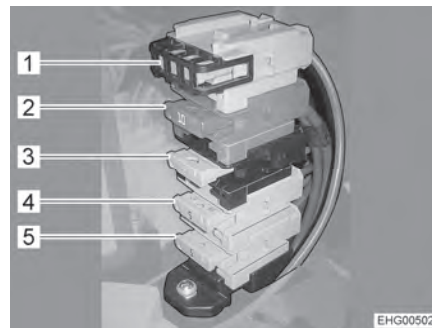
Fig. 105 Fusibles junto al bloque eléctrico con preparación para energía solar e instalación de antena parabólica
