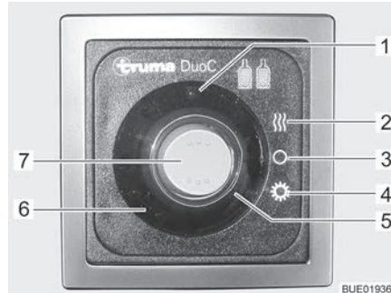
Afb. 45 Bedieningspaneel (DuoControl)
