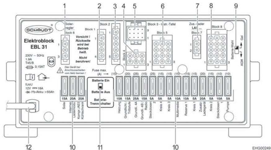
Afb. 49 Elektroblock (EBL 31)
