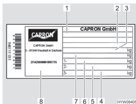
Afb. 87 Typeplaatje
