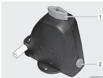
Afb. 72 Veiligheids-/aftapventiel geopend
