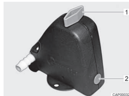
Afb. 73 Veiligheids-/aftapventiel gesloten
