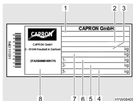
Fig. 131 Plaque signalétique
