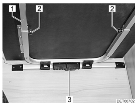
Fig. 40 Décaler/agrandir la table suspendue
