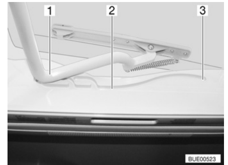
Fig. 37 Lanterneau Heki, glissière
