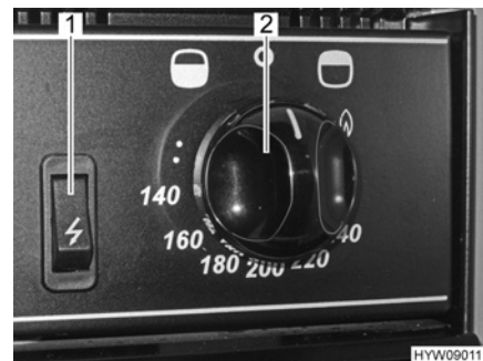
Fig. 93 Boutons de commande (four à gaz avec grill)
