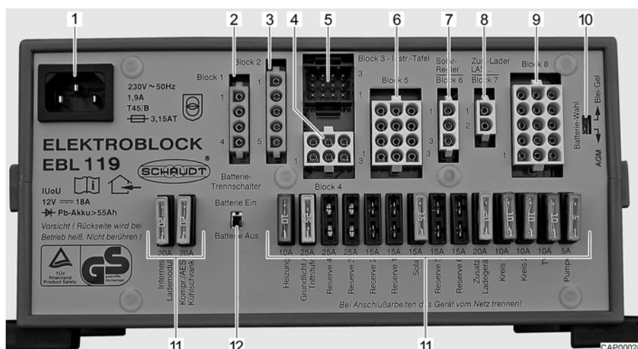
Fig. 71 Bloc électrique (EBL 119)
