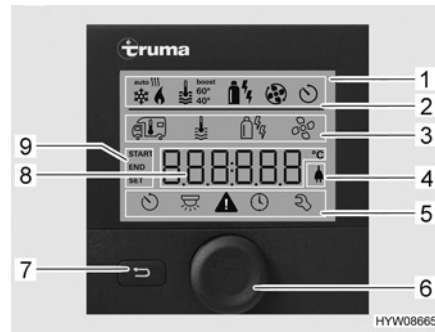
Fig. 85 Unité de commande avec affichages
