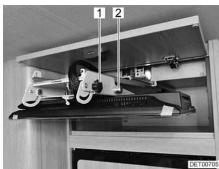
Fig. 45 Écran plat dans niche pour téléviseur
