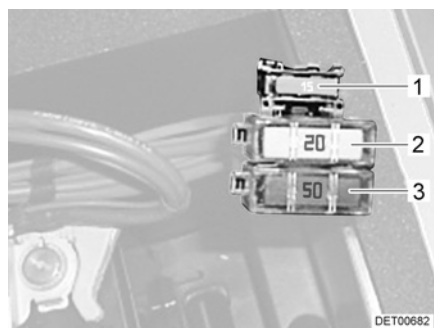
Fig. 76 Fusibles de la batterie de démarrage
