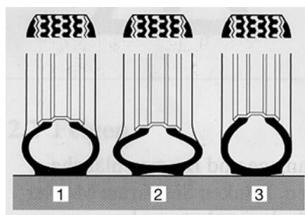
Fig. 133 Surface de contact du pneu
