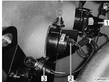
Fig. 123 Éclairage de l'avant (vue depuis le compartiment moteur)
