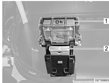
Fig. 77 Fusibles de la batterie de cellule
