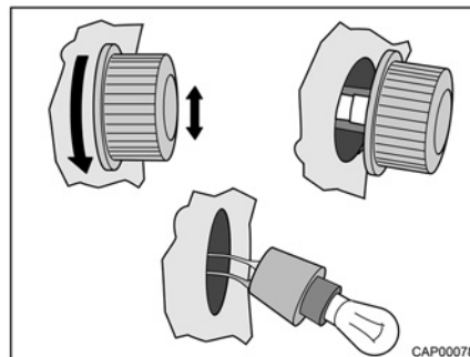
Fig. 124 Indicateur de direction latéral (12 V/5 W)
