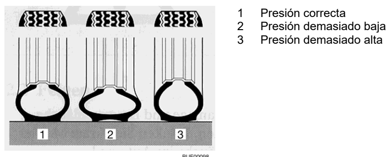
Fig. 144 Superficie de contacto del neumático
