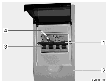
Fig. 86 Caja de fusibles de 230-V con interruptor de protección de línea y RCD (interruptor principal)
