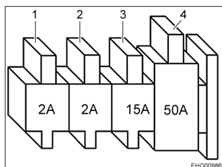
Fig. 92 Fusibles en la batería del motor de arranque
