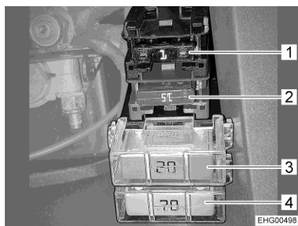
Fig. 91 Fusibles en la batería del motor de arranque con amplificador de carga
