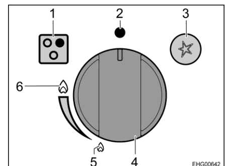
Fig. 108 Elementos de mando y de visualización
