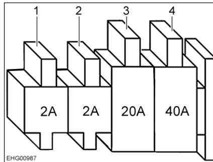
Fig. 95 Fusibles para dos baterías del habitáculo
