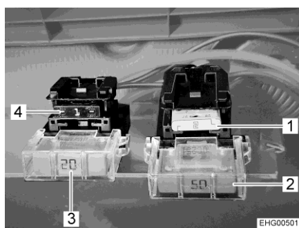
Fig. 93 Fusibles en la batería del habitáculo con amplificador de carga
