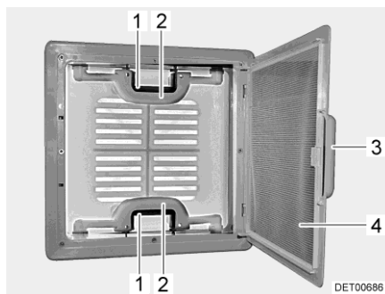
Fig. 31 Claraboya con cierre de resorte
