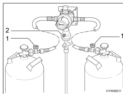
Fig. 8 Regulador de gas (DuoControl)
