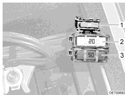
Fig. 90 Fusibles en la batería del motor de arranque sin amplificador de carga
