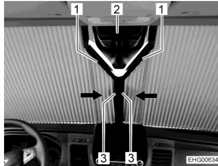
Fig. 30 Luna delantera con persianas plegables
