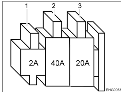
Fig. 94 Fusibles para una batería del habitáculo
