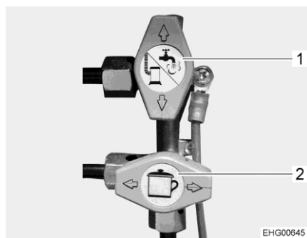
Fig. 100 Posición de las válvulas de paso de gas (ejemplo)
