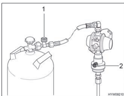
Bild 5 Gasregulator (MonoControl)
