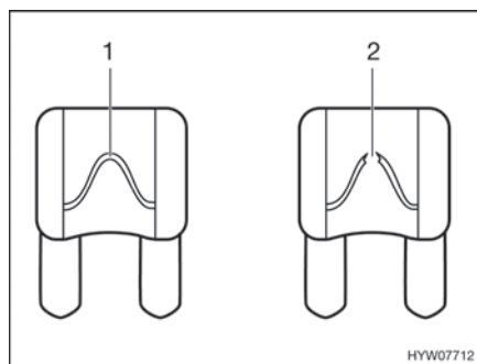
Bild 68 12 V-säkring
