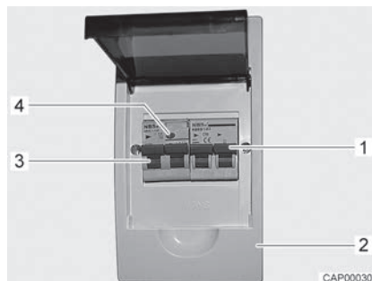
Bild 66 Ledningsskyddsbrytare och FI-brytare (230 V-säkringslåda)
