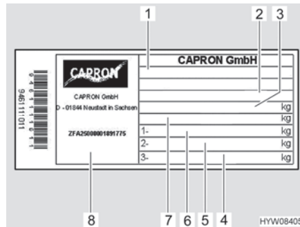
Bild 111 Typskylt
