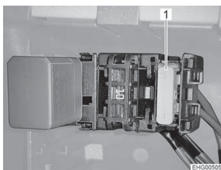
Bild 72 Säkring på B-stolpen, högra sidan av fordonet
