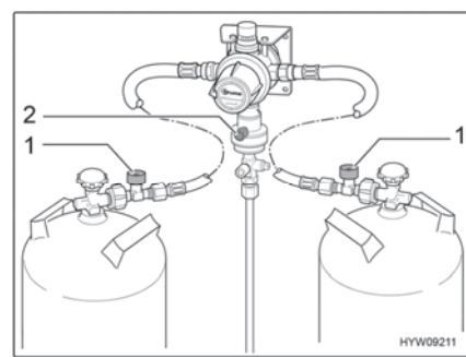
Bild 6 Gasregulator (DuoControl)
