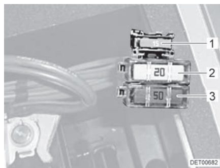
Bild 69 Säkringar vid startbatteriet utan laddningsbooster
