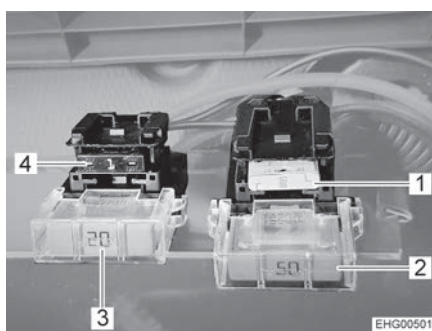
Bild 71 Säkringar vid bodelsbatteriet med laddningsbooster
