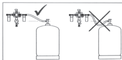
Bild 60 Korrekt anslutning av gasflaskan
