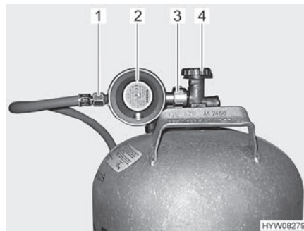
Bild 61 Anslutning gasflaska
