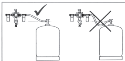
Afb. 51 Correcte aansluiting van de gasfles
