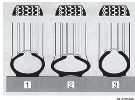
Afb. 95 Draagvlak van de band
