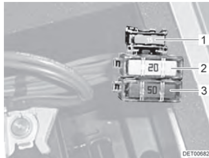
Afb. 59 Zekeringen aan de startaccu
