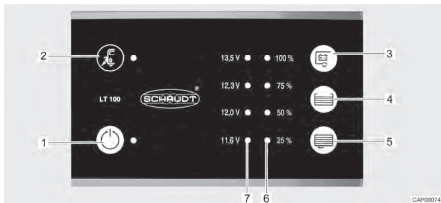
Afb. 55 Paneel (LT 100)
