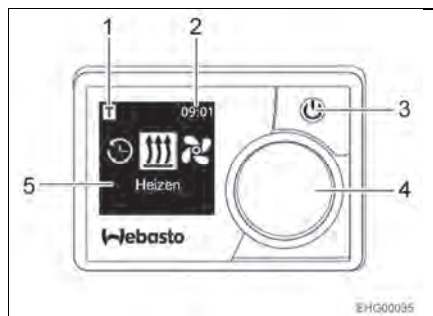
Afb. 66 Bedieningspaneel (standverwarming)
