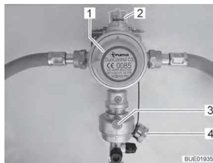
Afb. 49 DuoControl-regelaar
