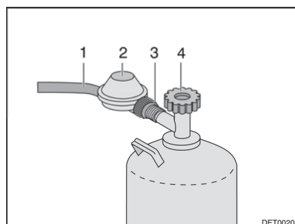
Kuva 91 Kaasupullon liittämä
