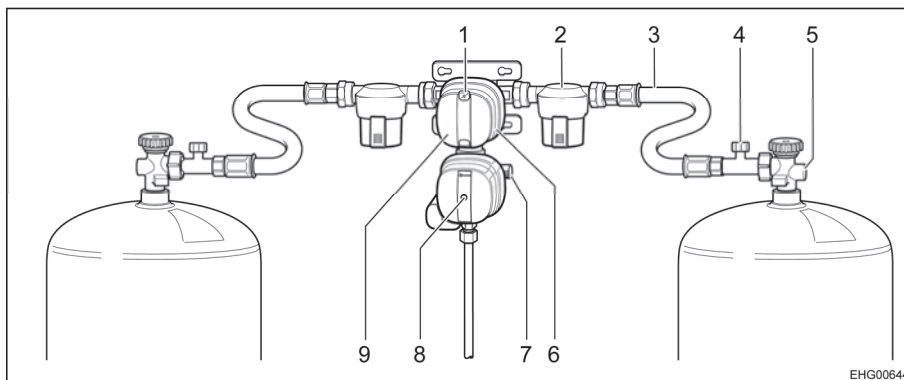
Bilde 69 Gasstrykk-kontrollsystem DuoControl CS
