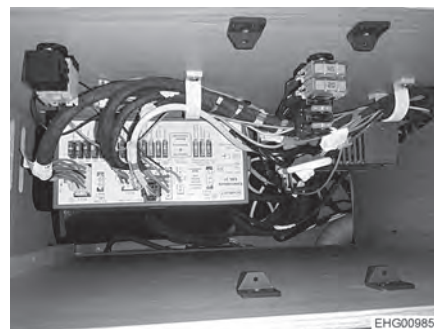
Bilde 75 Monteringssted for strømsentralen (Ford)
