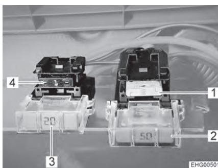
Bilde 84 Sikringer ved boenhetsbatteri med Lade-Booster
