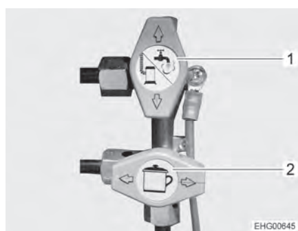
Bilde 91 Posisjon gassavstengeventiler (eksempel)
