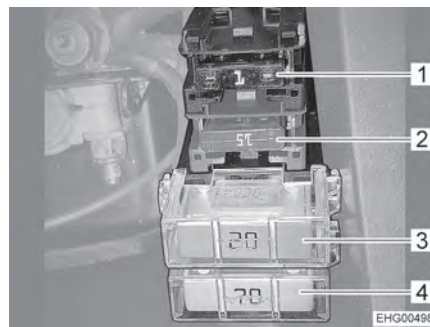
Bilde 82 Sikringer ved startbatteriet med lade-booster
