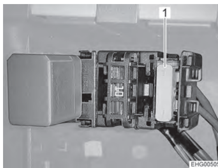
Bilde 87 Sikring på B-søyle, høyre kjøretøyside
