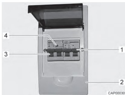
Bilde 78 Ledningsbeskyttelsesbryter og FI-bryter (230 V-sikringsboks)
