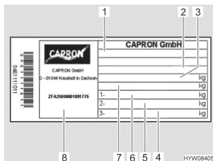
Bilde 1 Typegodkjenningsskilt
