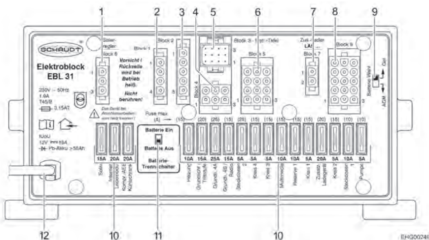
Bilde 76 Strømsentral (EBL 31)
