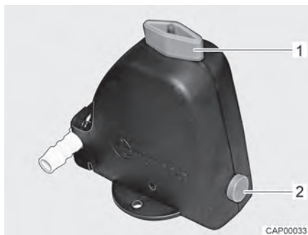
Bilde 105 Sikkerhets-/avtappingsventil åpnet
