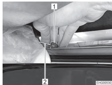
Bilde 58 Nødopplåsing
