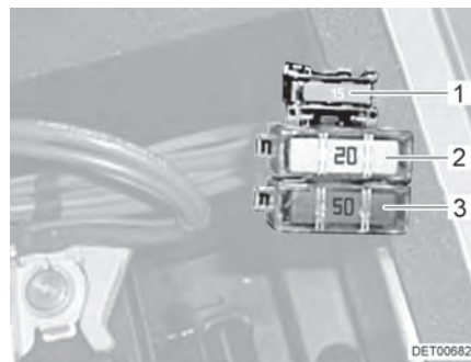
Bilde 81 Sikringer ved startbatteriet uten Lade-Booster
