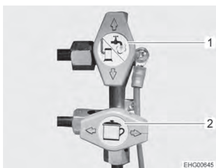
Bilde 73 Gassavstengeventiler
