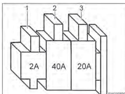
Bilde 85 Sikringer hvis man har et boenhets-batteri
