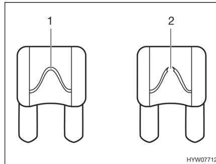
Bilde 80 Sikring 12 V
