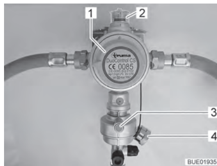
Bilde 68 DuoControl-kontrollsystem
