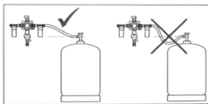
Bilde 71 Riktig tilkobling av gassflasken
