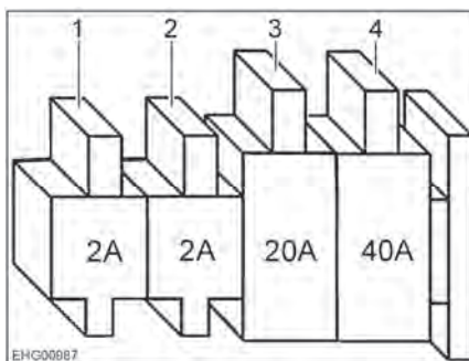
Bilde 86 Sikringer hvis man har to boenhets-batterier
