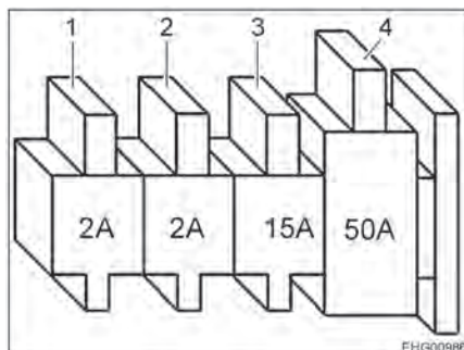
Bilde 83 Sikringer ved startbatteriet
