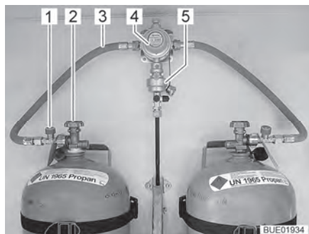
Bilde 67 Gassflasker med DuoControl
