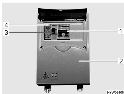
Fig. 70 Caja de fusibles de 230 V con interruptor de protección de línea e interruptor FI
