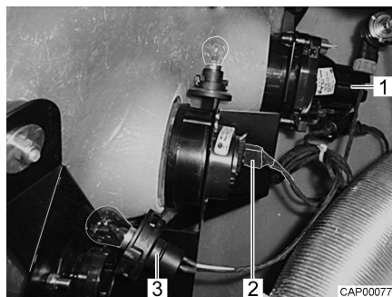
Fig. 119 Iluminación del frente (vista desde el compartimento del motor)
