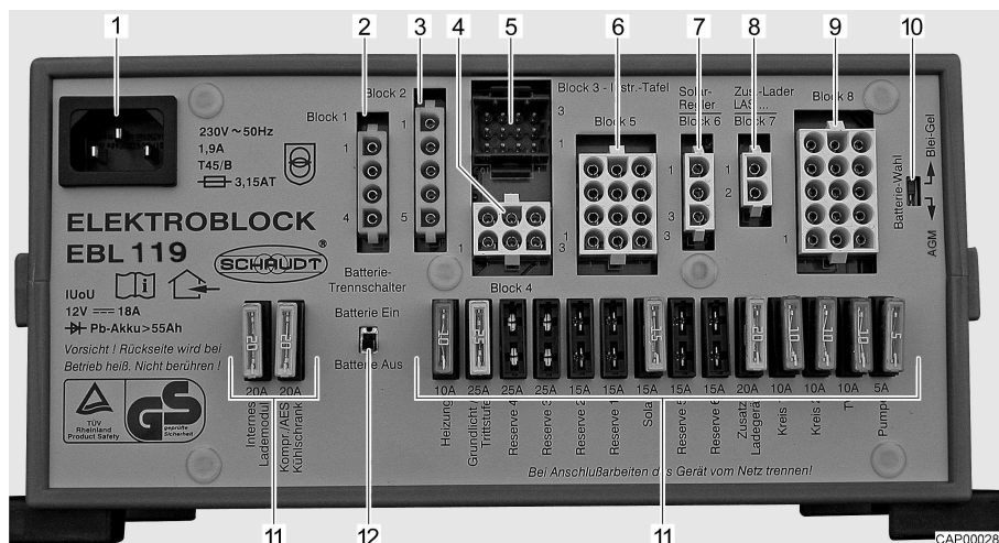
Fig. 68 Bloque eléctrico (EBL 119)
