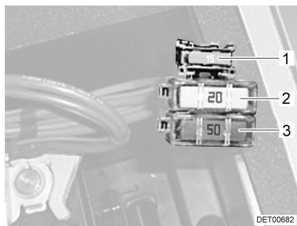
Fig. 73 Fusibles en la batería del motor de arranque
