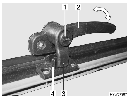
Fig. 21 Palanca de bloqueo en la posición de "cerrado"
