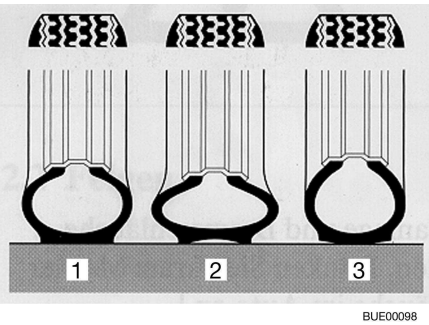
Fig. 129 Superficie de contacto del neumático
