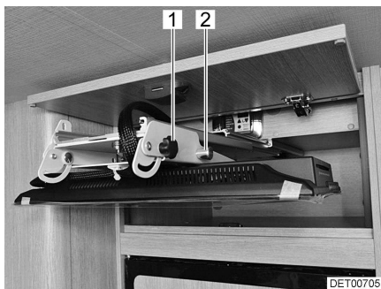
Fig. 43 Pantalla plana en el compartimento de televisor
