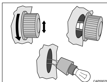
Fig. 120 Intermitente lateral (12 V/5 W)
