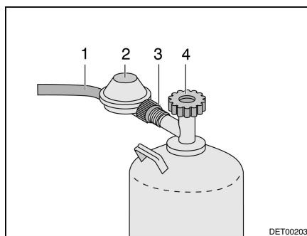
Fig. 65 Conexión de la bombonas de gas
