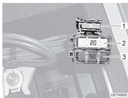
Fig. 85 Fusibles de la batterie de démarrage
