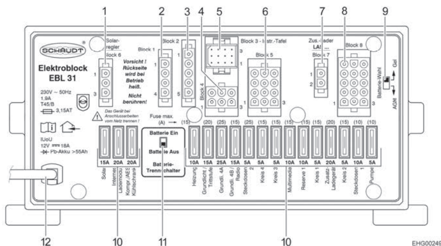
Fig. 80 Bloc électrique (EBL 31)
