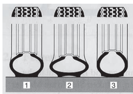
Fig. 141 Surface de contact du pneu
