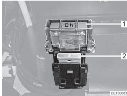
Fig. 86 Fusibles de la batterie de cellule
