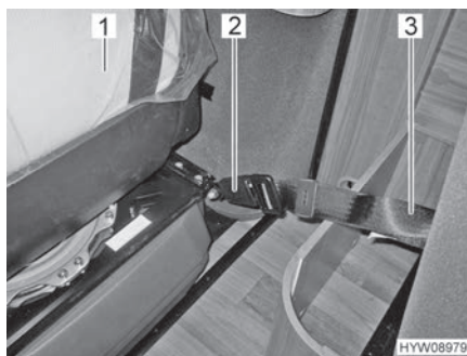
Fig. 15 Bloquer le siège emboîtable avec la boucle de fermeture de la ceinture
