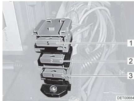
Fig. 87 Fusibles à côté du bloc électrique
