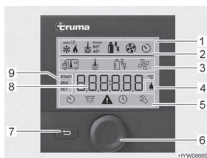
Fig. 94 Unité de commande avec affichages
