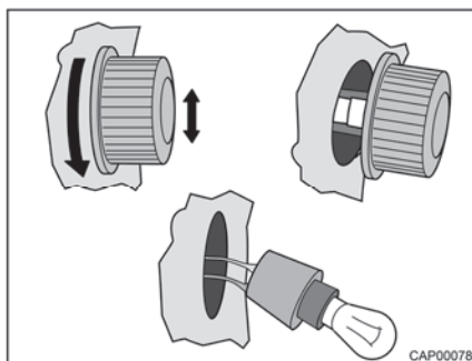
Fig. 132 Indicateur de direction latéral (12 V/5 W)
