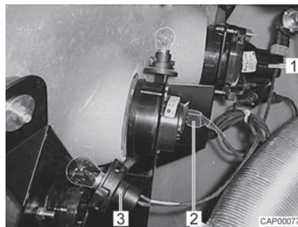
Fig. 131 Éclairage de l'avant (vue depuis le compartiment moteur)
