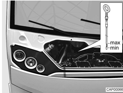
Kuva 8 Öljynmittatikku (moottoriöljy)
