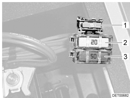
Kuva 73 Sulakkeet käynnistysakun luona
