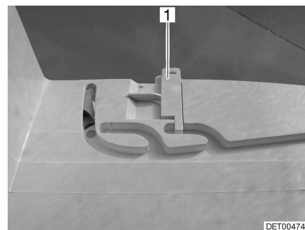
Kuva 37 Tuuletusasennon lukitus
