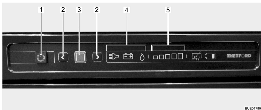
Kuva 93 Jääkaapin käyttölaitteet
