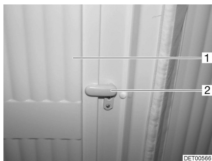
Kuva 108 Salpaus, WC-tilan verhous
