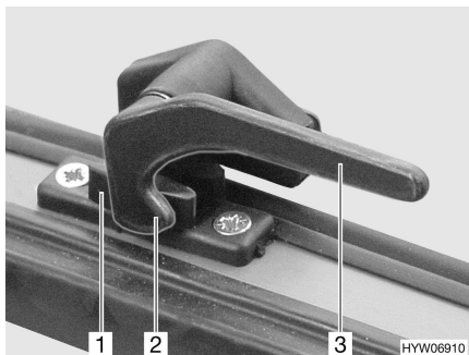
Kuva 27 Lukitusvipu asennossa "kiinni"
