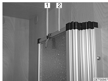
Kuva 109 Kiinnitys, suihkuseinä
