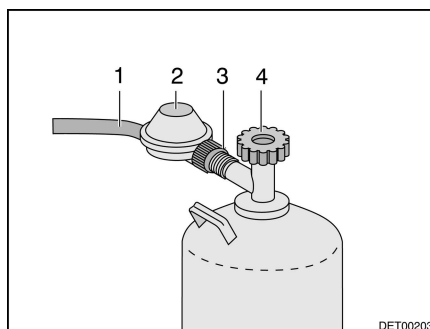
Kuva 65 Kaasupullon liitäntä
