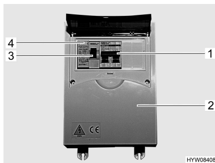
Kuva 70 230 V:n sulakerasia ja johdinsuojakytkin sekä FI-kytkin
