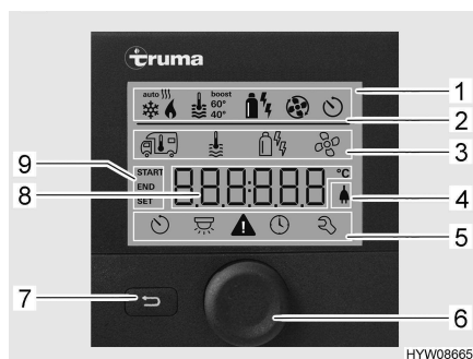
Kuva 82 Säätöyksikkö näytöillä
