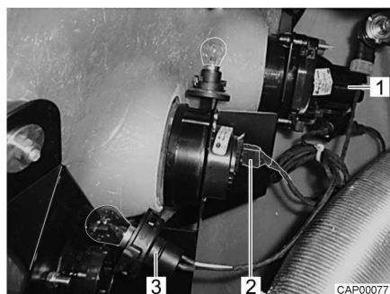
Kuva 119 Etuvalaistus (näköymä moottorin kautta)
