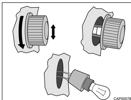
Kuva 120 Sivusuuntavilkku (12 V/5 W)
