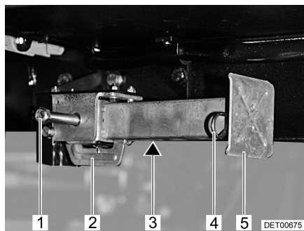
Kuva 14 Nostotuki
