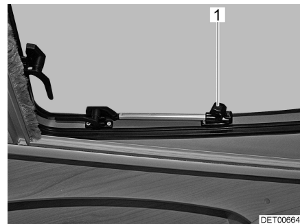
Kuva 28 Kattoikkuna, jossa on kääntöpidikkeet, avattu
