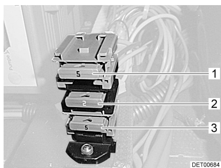
Kuva 75 Sähkö- ja elektroniikkayksikön vieressä olevat sulakkeet
