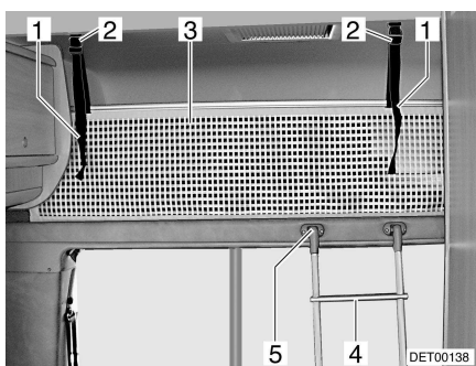
Kuva 47 Alkovivuode
