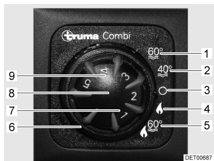
Kuva 80 Säätyyksikkö
