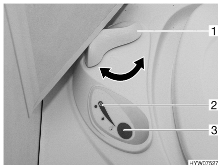
Kuva 112 Thetford-WC:n säätöyksikkö
