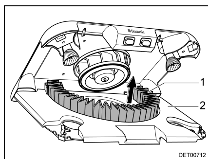
Kuva 117 Aktiivihiihisuodattimen vaihtaminen
