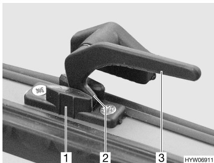
Kuva 29 Lukitusvipu asennossa "jatkuva tuuletus"
